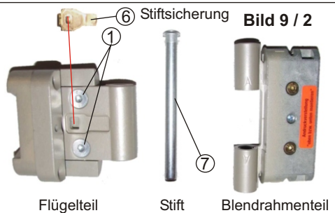
Flügelteil
